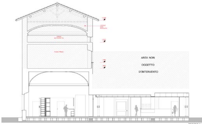
SEZIONE A-A
